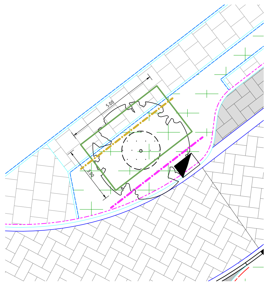
PRINCIPE DETAIL: PLANTVAK LANGS RIJBAAN (2) SCHAAL 1:100
