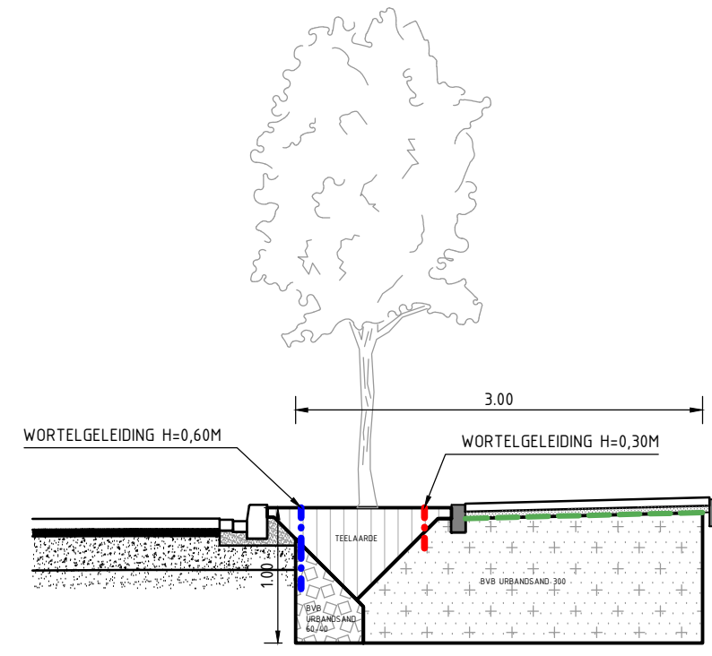
PRINCIPE DETAIL: PLANTVAK LANGS RIJBAAN (1) SCHAAL 150
