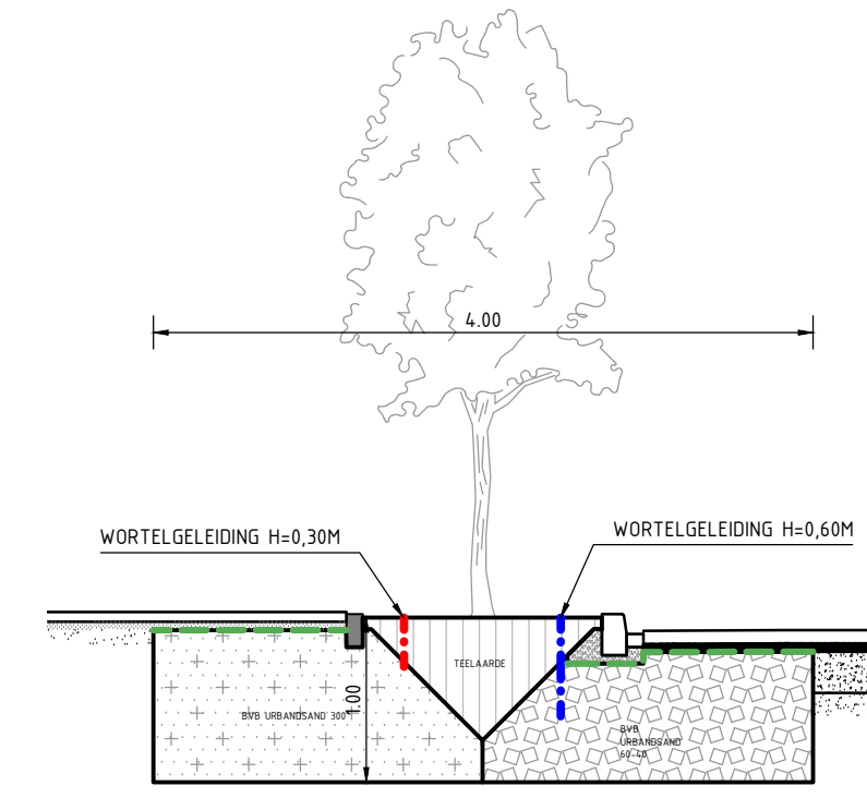
PRINCIPE DETAIL: PLANTVAK LANGS HAAKSPARKEREN SCHAAL 150
