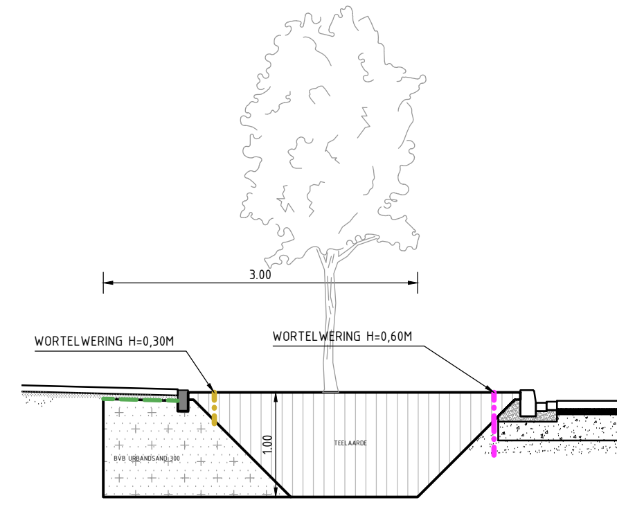
PRINCIPE DETAIL: PLANTVAK LANGS RIJBAAN (2) SCHAAL 150
