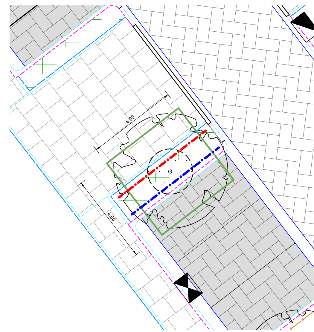
PRINCIPE DETAIL: PLANTVAK LANGS HAAKSPARKEREN SCHAAL 1:100
