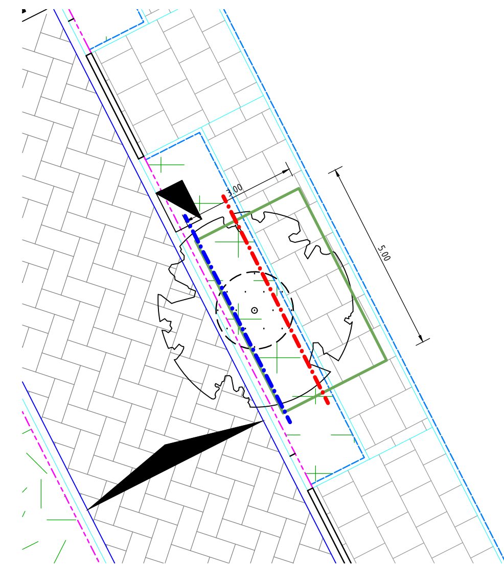
PRINCIPE DETAIL: PLANTVAK LANGS RIJBAAN (1) SCHAAL 1:100
